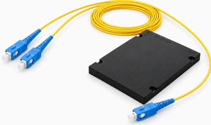
DIVISOR ÓPTICO PLC EN CAJA 1x2 SC/UPC · 1260-1650 nm
