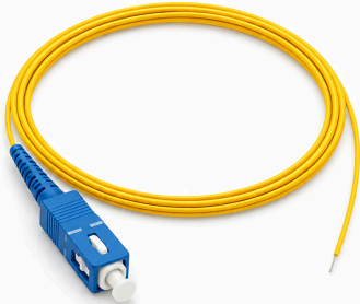
PIGTAIL DE FIBRA ÓPTICA OS2 monomodo 9/125 \mu\text{m} SC/UPC Longitud 1.5 m · Carrier-grade
