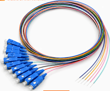
KIT DE 12 PIGTAILS OS2 MONOMODO SC/UPC 12 pigtails de 6.56 FT · OS2 monomodo 9/125 \mu\text{m}
