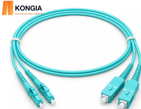
PATCH CORD DE FIBRA ÓPTICA 1 m · OM3 · Duplex LC/UPC ↔ SC/UPC LSZH · 2.0 mm · 2 fibras KG-FO-PC-LCU-SCU-OM3-DX-01M
