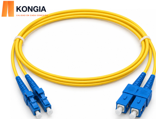
PATCH CORD DE FIBRA ÓPTICA 1 m · OS2 · Duplex LC/UPC ↔ SC/UPC LSZH · 2.0 mm · 2 fibras KG-FO-PC-LCU-SCU-OS2-DX-01M
