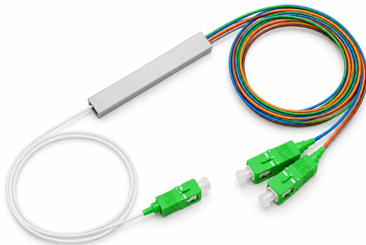
DIVISOR ÓPTICO PLC MINI 1x2 SC/APC · 1 m
