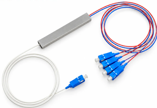
DIVISOR ÓPTICO PLC MINI 1x4 SC/UPC · 1,0 m
