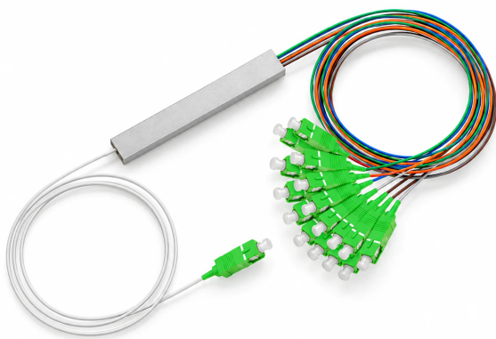
DIVISOR ÓPTICO PLC MINI 1x8 SC/APC · 1,0 m
