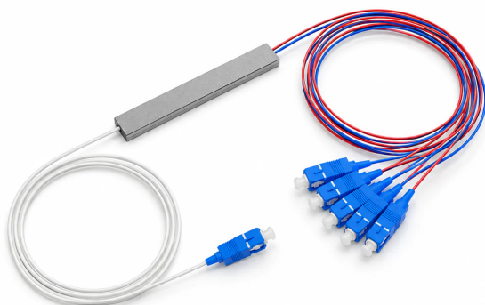
DIVISOR ÓPTICO PLC MINI 1x8 SC/UPC · 1,0 m
