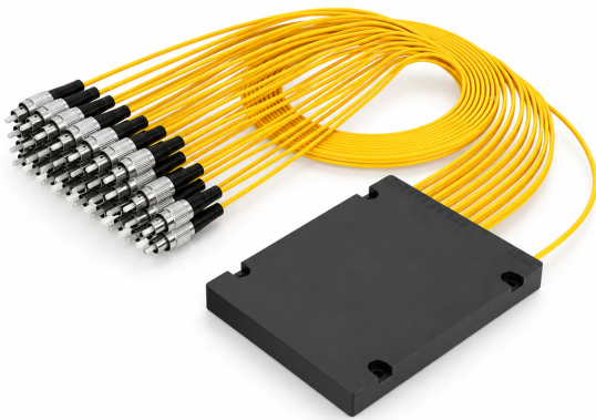
DIVISOR ÓPTICO PLC EN CAJA 1×16 FC/UPC · 1260–1650 nm
