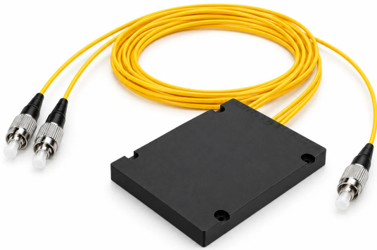
DIVISOR ÓPTICO PLC EN CAJA 1x2 FC/UPC · 1260-1650 nm
