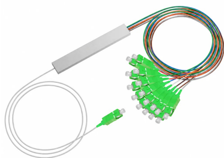
PLC mini 1x4 · SC/APC KG-FO-PLC-1X4-APC Imagen de referencia de la serie
