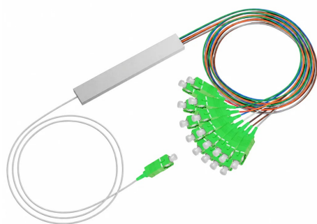
PLC mini 1x8 · SC/APC KG-FO-PLC-1X8-APC Imagen de referencia de la serie
